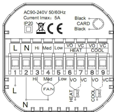
Klemmenbelegung Rückseite
